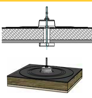
Dakplaat Hout – Tuimelanker
