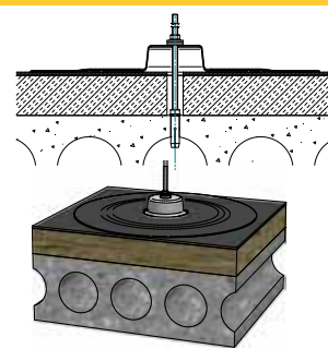
Kanaalplaatvloer – Mechanisch Anker
