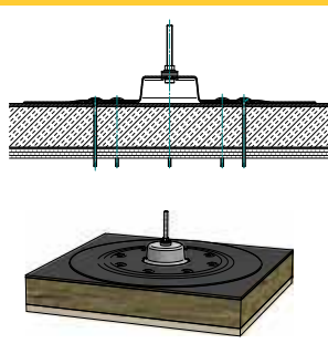
Dakplaat Hout – Schroeven
