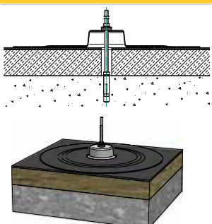
Volbeton dakvloer – Mechanisch Anker
