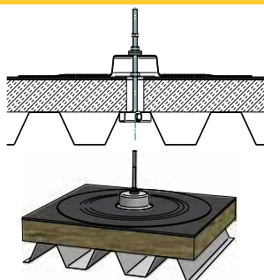
Dakplaat Metaal – Tuimelanker
