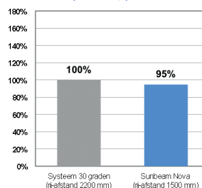
Rendement (kWh/kWp)
